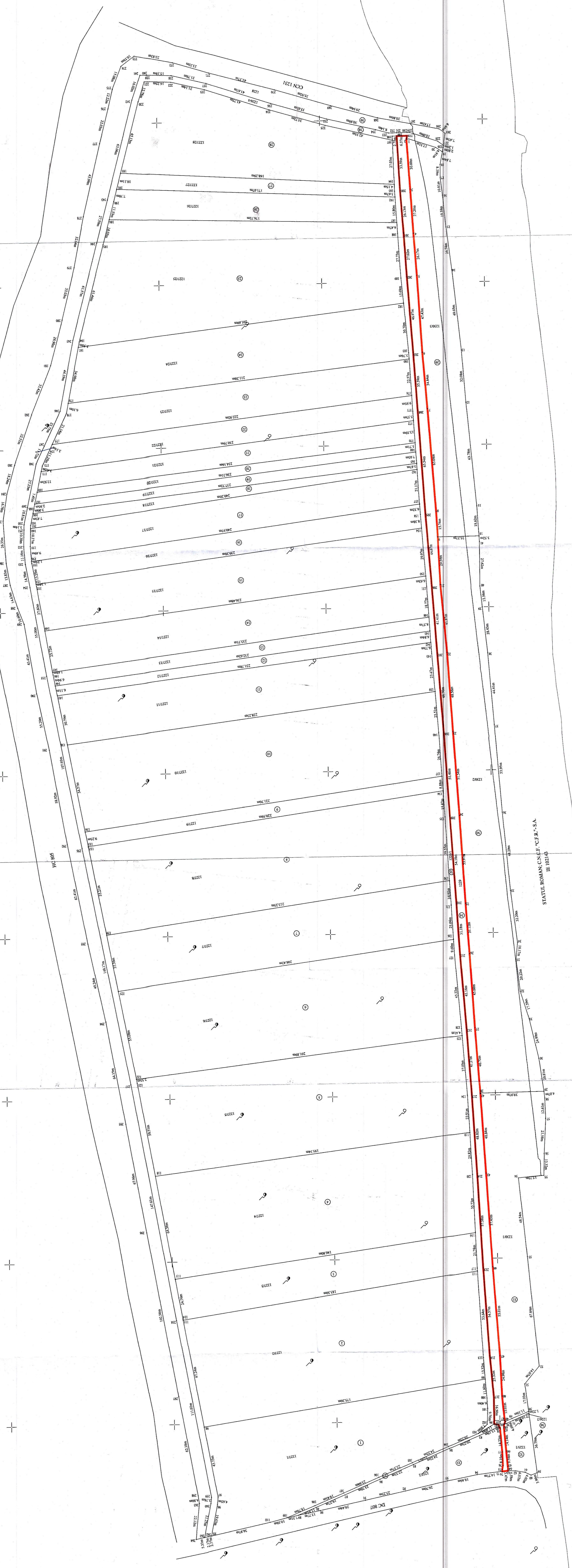
PLAN PARCELAR Scara 1:1000 Comuna: Cata, Judetul Brasov Taria 71 - A1227, A1230, A1225 Sistem de protectie Stereografica 1970
